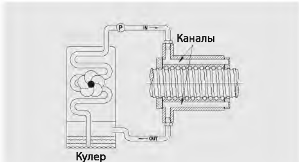
Рис. 9.2 Гайка с охлаждением тип 1 (Cool type I) и кулер.
