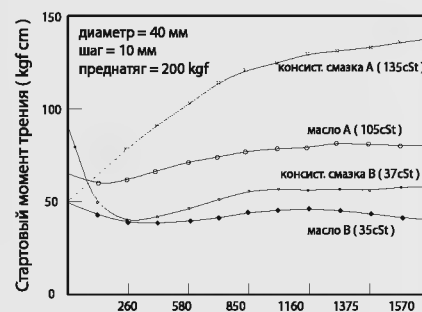
Рис 4.31 Влияние вязкости смазки на момент трения
