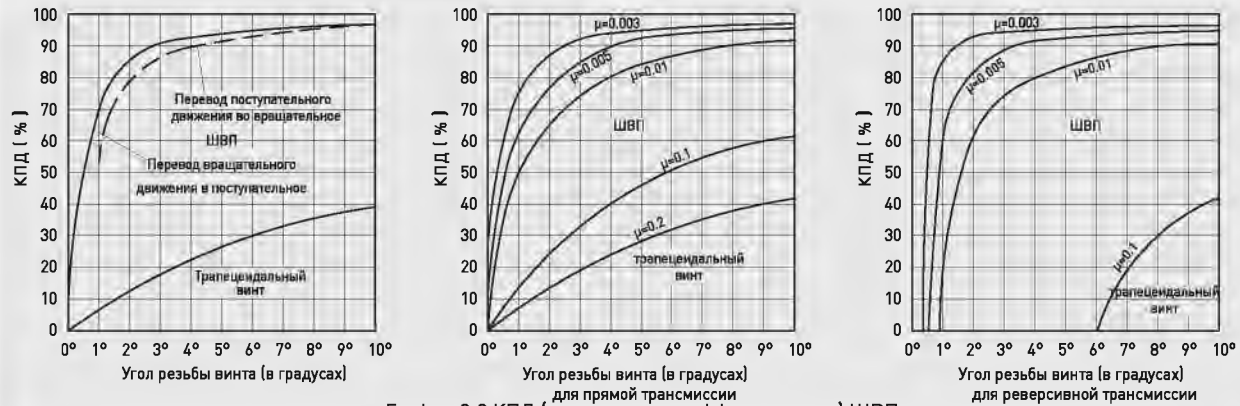
График 2.2 КПД (механическая эффективность) ШВП
