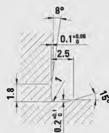
F1X0.2DIN509
