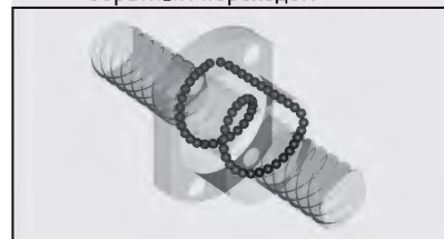
Рис. 3.3 Внутренний тип рециркуляции шариков с концевой системой возврата
