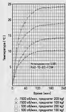
Рис 4.29 Связь рабочей скорости, преднатяга и рост температуры
