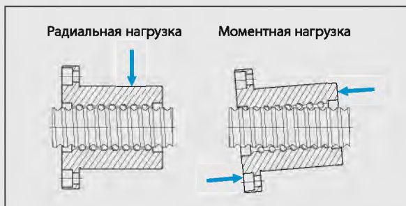
Рис 4.2(a) Дисбаланс в системе вызванный несоосностью её элементов: подшипниковых опор и гайки ШВП проблемы с корпусом гайки и т.д.
