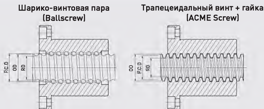
Рис 2.1 Базовое строение шарико-винтовой пары и трапецеидального винта с гайкой (ACME Screw)
